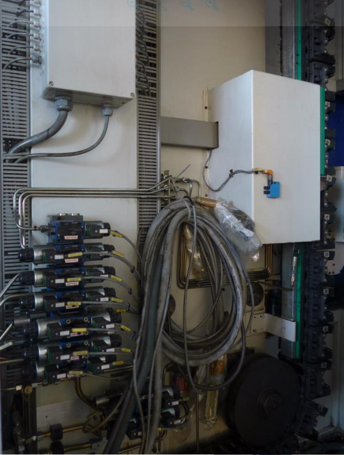
Werkzeugkettenwechsler Mit 50 Werkzeugplätzen
