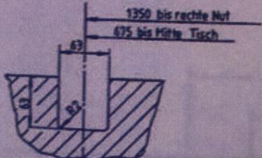
Nute für Werkzeugwechsel
