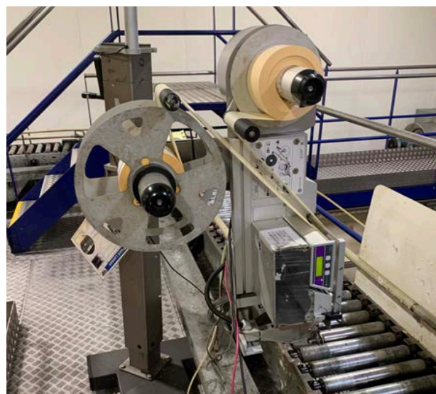
Markem Pack Labeller
