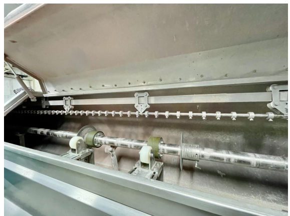
3.- Stripping nozzle detail
