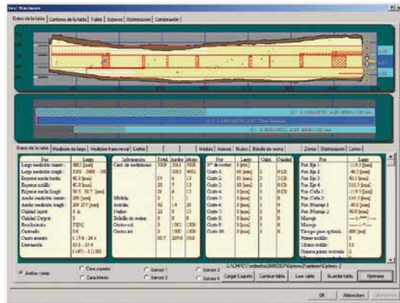
Anzeige des Optimierungsergebnisses für das Brett, mit Brettkontur, Lage und Abmessung der Produkte
