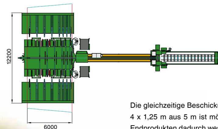
Optimes Line – BKO mit Beschickungssystem von beiden Seiten
