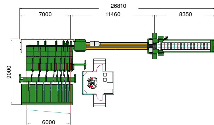
Optimes Line – BKO mit Beschickungssystem von rechts
