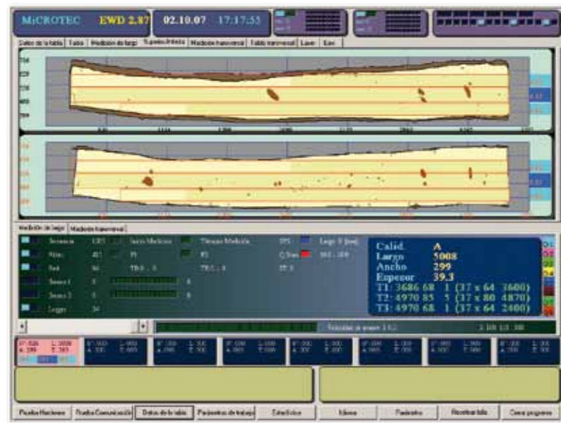
Brettober- und Brettunterseite mit der Lage der Produkte, der Besäum- und Trennschnitte und der Produktlängen
