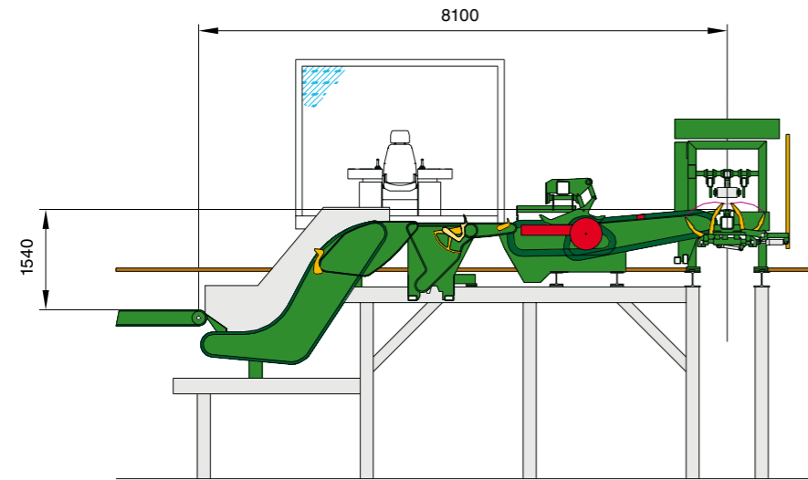
Optimes Line – BKO mit Beschickungssystem von rechts
