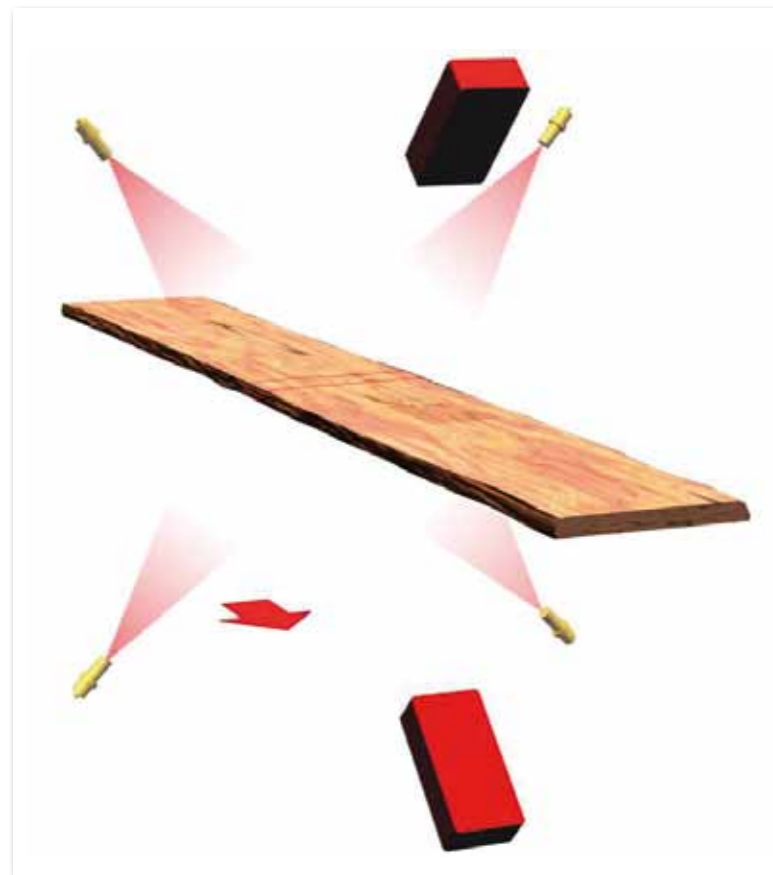
4-Kanten-Brettmeßsystem
