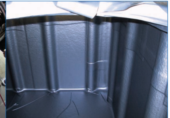
Einbau von Kunststoffinnenhüllen / Leckschutzauskleidungen inkl. Leckanzeiger
